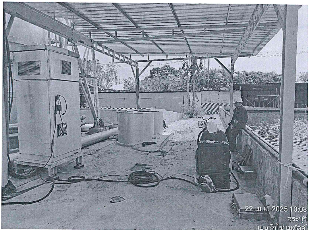
ปล่อยระบายจากเตาหลอมอาคาร 1 (โรงกรองอากาศ 7)
