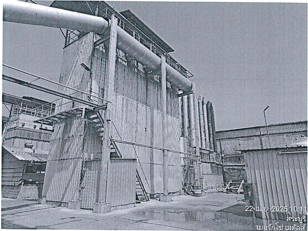
ระบบบำบัดของปล่องระบายจากเตาหลอมอาคาร 1 (โรงกรองอากาศ 6)
